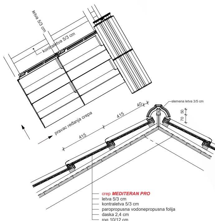
DETALJI POKRIVANJA SLEMENA KROVA
